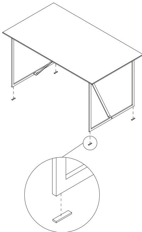
(d) Feltro adesivo rettangolare Rectangular adhesive felts
